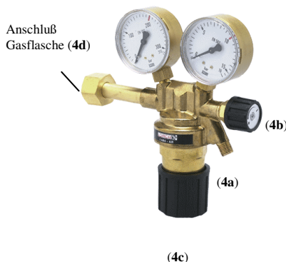
SPEIDEL-Druckminderer (4)
